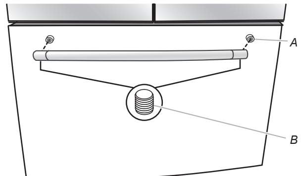
A. Tornillos de hombro B. Tornillos de fijación dentro del mango
