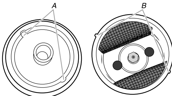
A. Fentes du chapeau du brûleur B. Onglets de la base du brûleur
