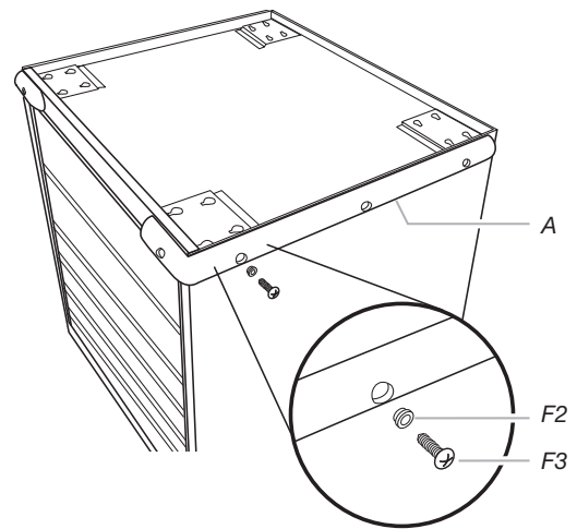
A. Bumper
