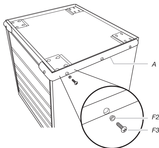
A. Butoir
