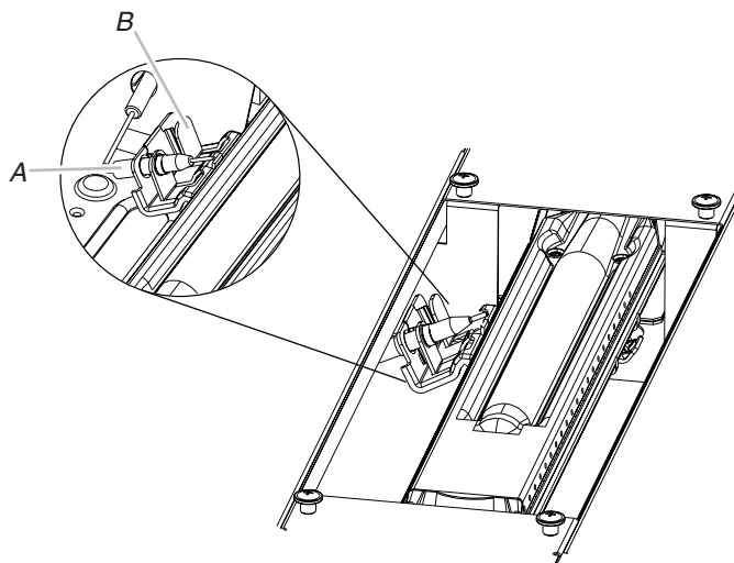
A. Electrodo del quemador para hornear del horno
