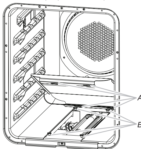
A. Orificios de montaje (chaveteros) de los tornillos de tope
