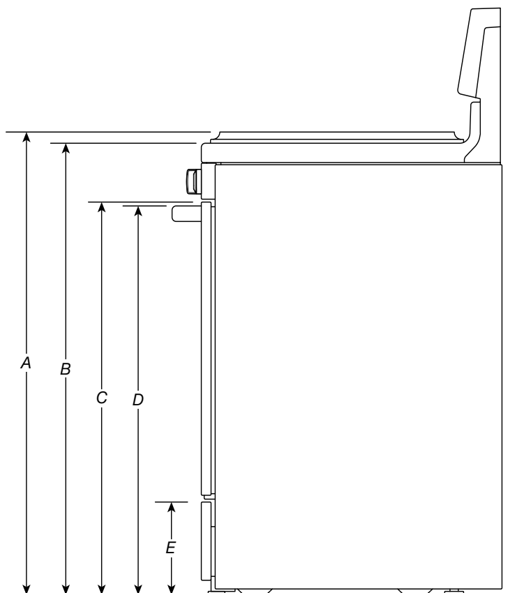
VUE LATÉRALE
