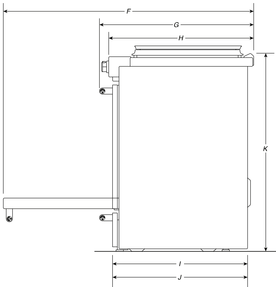
VUE LATÉRALE
