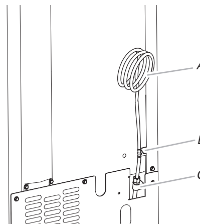
A. Tube en cuivre B. Bride du tuyau du robinet C. Bride de tuyau d'entrée d'eau et raccord de canalisation
