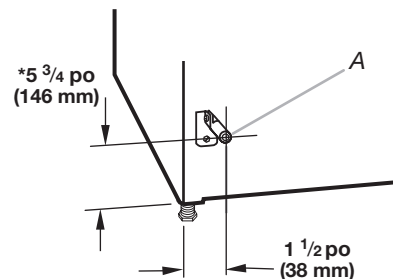
A. Conduit NPT de la sècheuse de 3/8 po
