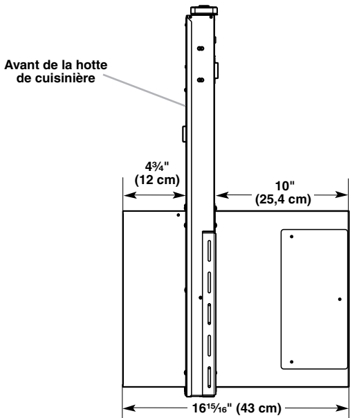
Ventilateur inversé
