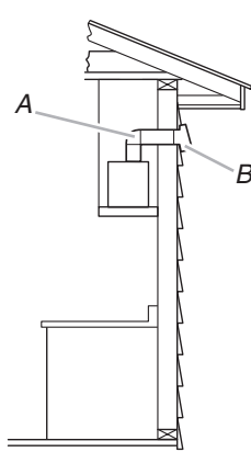
A. Conduit de dia. 6" (15,2 cm) pour décharge à travers le mur B. Bouche de décharge murale
