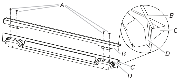
A. Vis n° 8-18 x 1/4" (6,4 mm) C. Pièce d'évent supérieure B. Déflecteur du tiroir-réchaud D. Pièce d'évent inférieure
