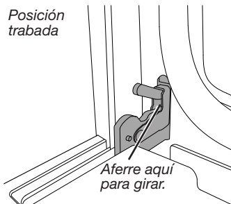
A. Traba de bisagra de la puerta del horno en posición trabada
