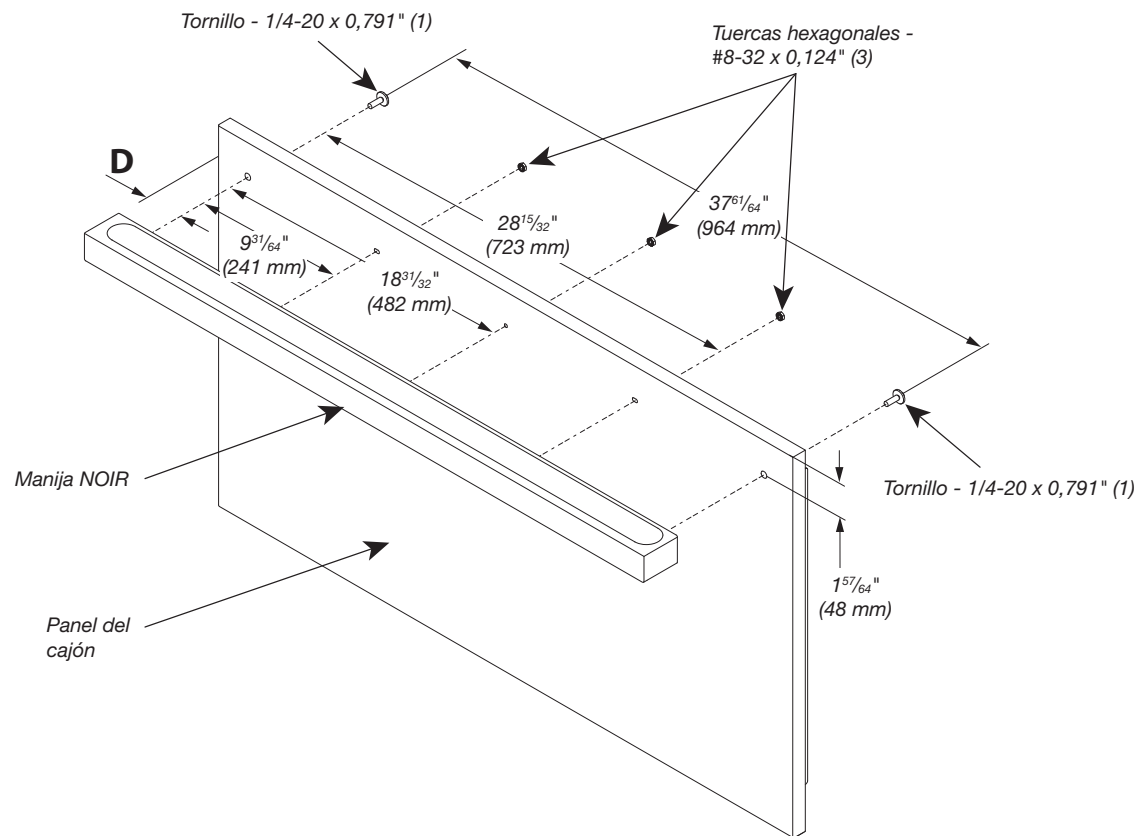
Figura 4 - 42" Cajón del congelador para montaje inferior en puerta francesa
