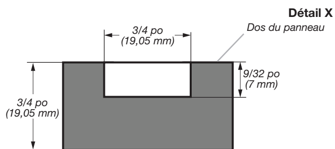
Illustration 5 – Vue transversale
