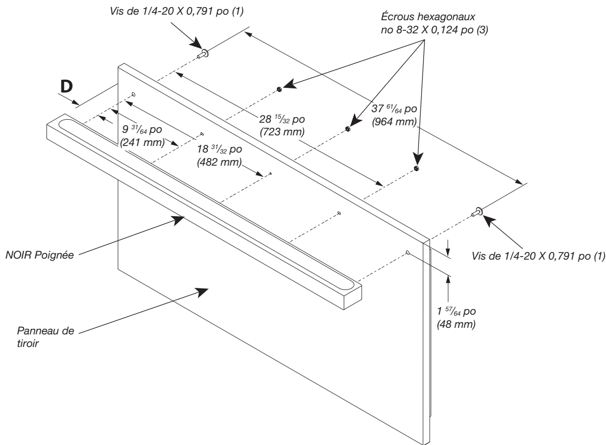
Illustration 4 – Modèles de 42 po avec porte double et tiroir de congélateur en bas
