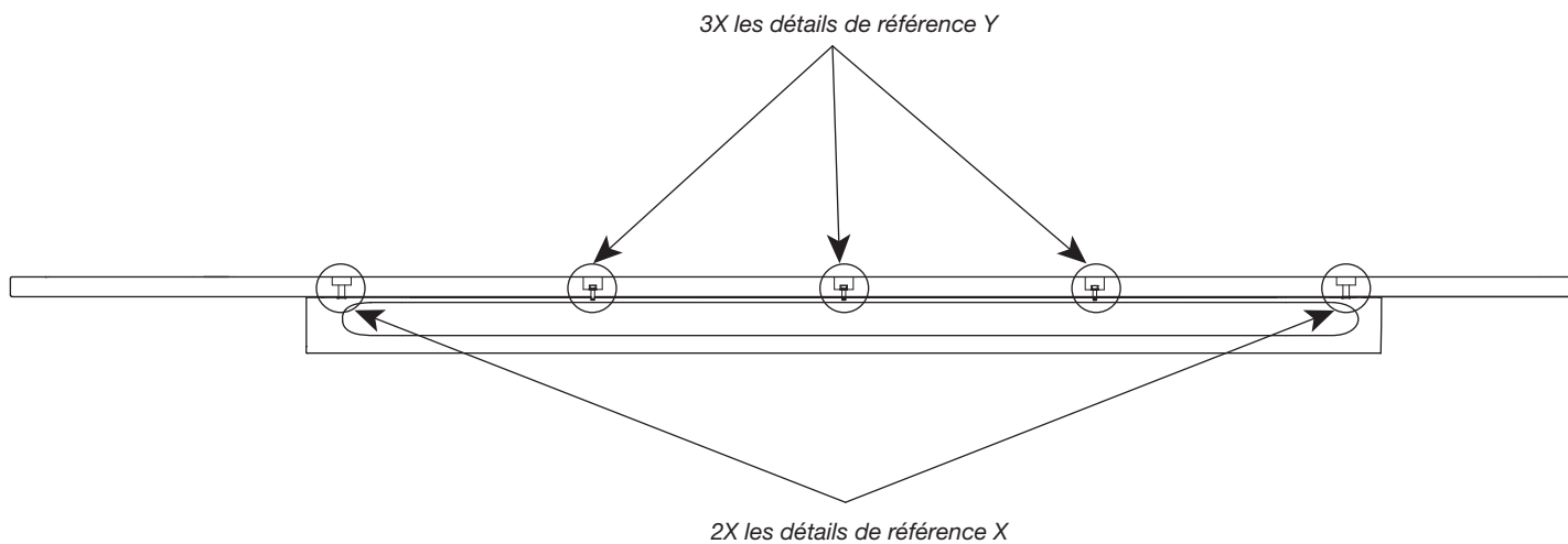
Illustration 5 – Vue transversale
