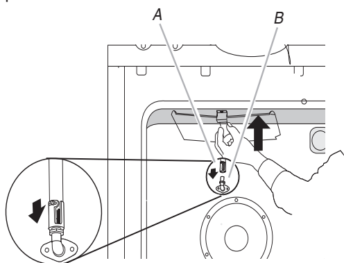
A. Gicleur de brûleur de gril B. Grille de la lèche-frite
