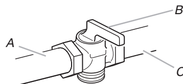
A. Vers la cuisinière B. Robinet d'arrêt (position de fermeture) C. Canalisations d'alimentation en gaz
