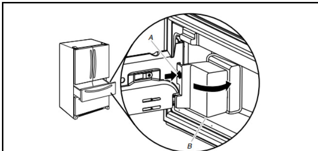
A. Lengüeta de cubierta B. Cubierta de conexión de cableado
