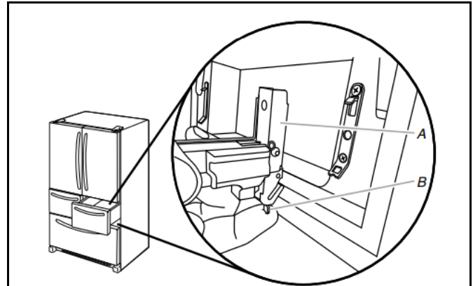
A. Soporte de la guía del cajón B. Palanca de liberación
