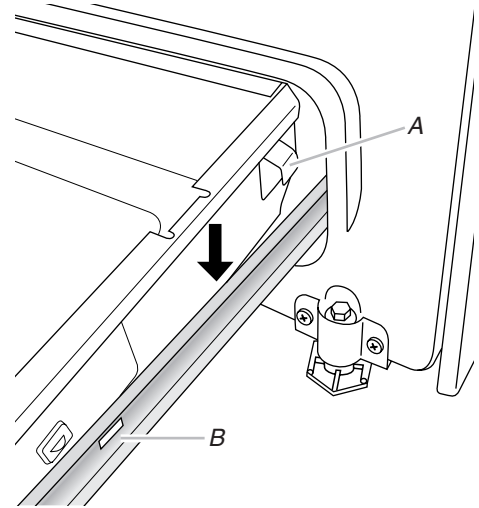
A. Lengüeta de alineación del cajón B. Muesca de la guía del cajón
