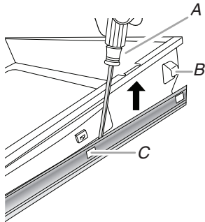
A. Destornillador de hoja plana B. Lengüeta de alineación del cajón C. Muesca de la guía del cajón
