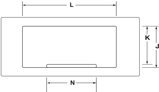
VUE AVANT INTÉRIEURE DE LA CAVITÉ
