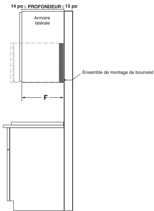
VUE LATÉRALE
