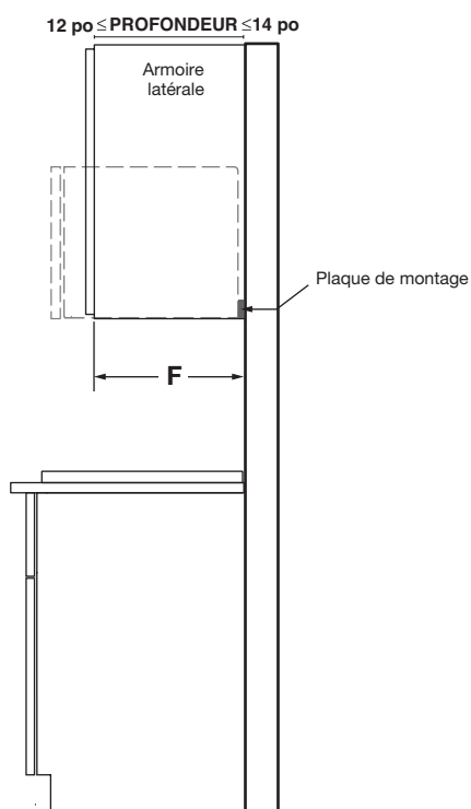
VUE LATÉRALE
