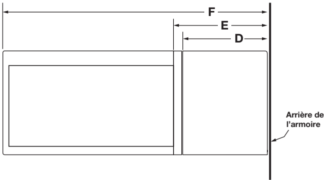
VUE LATÉRALE
