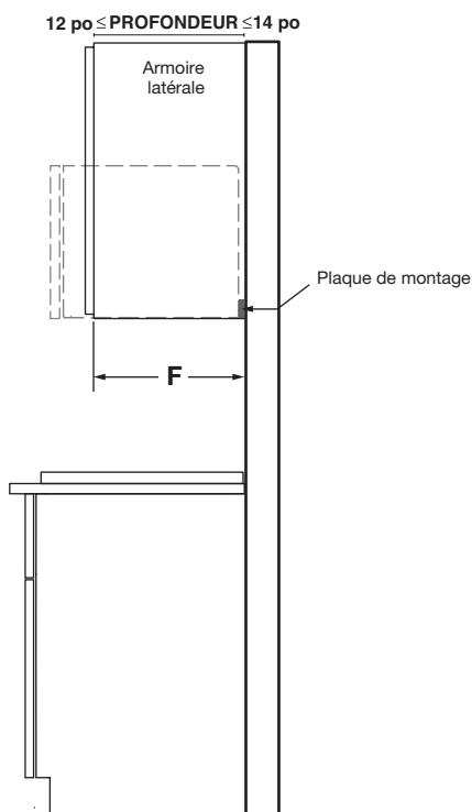
VUE LATÉRALE
