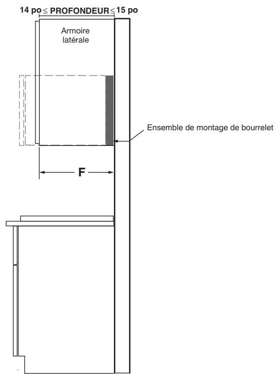
VUE LATÉRALE
